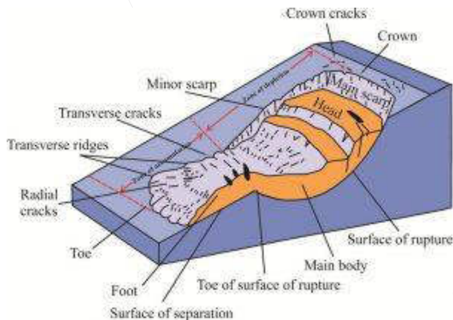
Slika 2. Elementi klizišta
